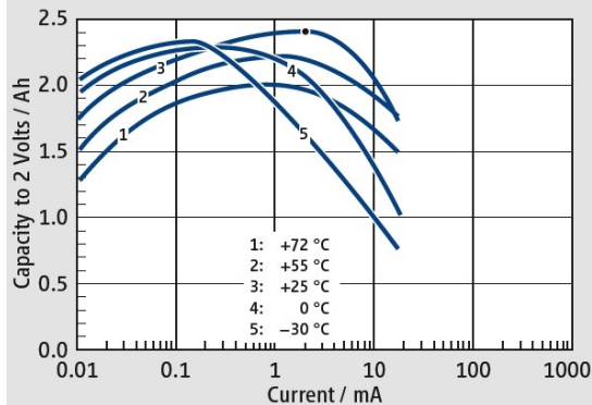
Pojemność / Prąd
