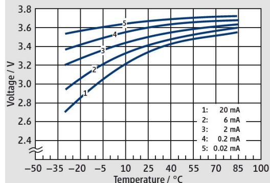
Napięcie / Temperatura
